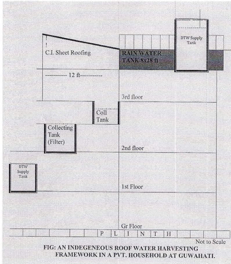
चित्र-3-गुवाहाटी के एक निजी मकान में छत पर जल संचयन का स्वदेशी ढ़ंचा सीआई शीट रूफिंग, डीटीडब्ल्यू आपूर्ति टक, 12 फुट , तीसरी मंजिल, दूसरी मंजिल, पहली मंजिल कूल टक, संग्रहण टक, डीटीडब्ल्यू आपूर्ति टक, ग्राउंड फ्लोर (पाइप) (स्केल पर नहीं है)
